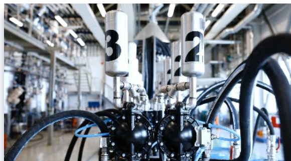
Автоматическое дозирование жидких добавок
